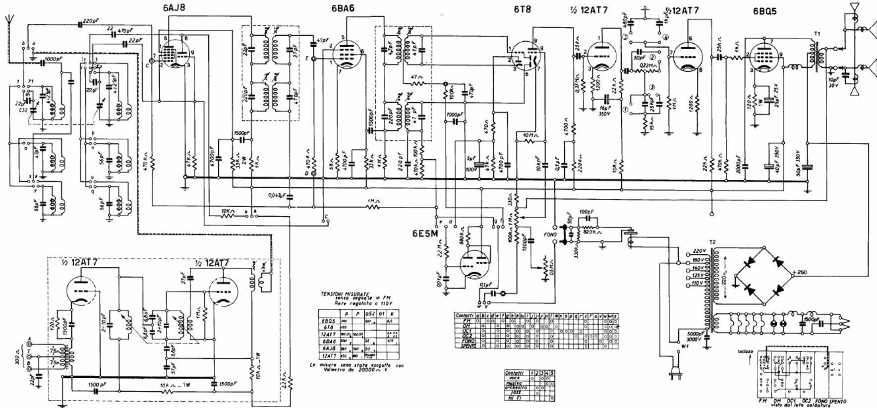
IMCARADIO - Mod. IF 77/B. Apparecchio AM/FM con una gamma onde medie, due gamme onde corte e una gamma ultracorte a modulazione di frequenza. Riproduzione sonora ad alta fedeltà con quattro altoparlanti. Media frequenza a 460 kc/s. Regolatore toni a cinque contatti. Potenza indistorta d'uscita 3,5 watt. Consumo medio 50 watt.
